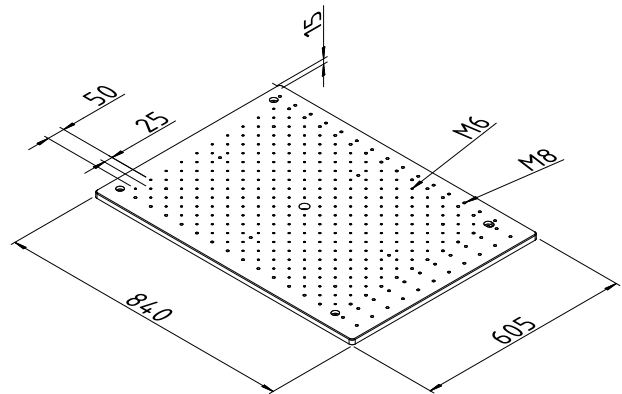
taban plakası K551187 CMM CRYSTA-Apex S574 için
