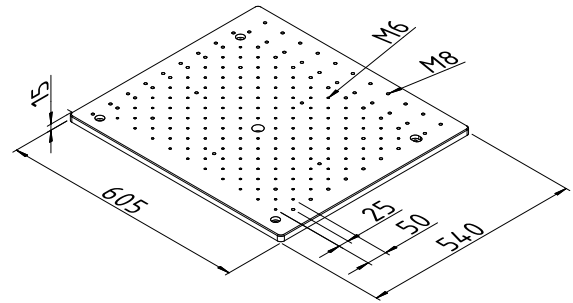
taban plakası K551186 CMM CRYSTA-Apex S544 için
