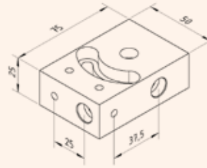
Parça No.: K551121 Ağırlık 200 g
