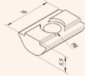
Parça No.: K551158 Ağırlık 5 g
