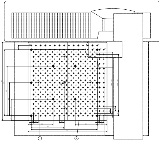
taban plakası K551190 CMM CRYSTA-Apex S776 için
