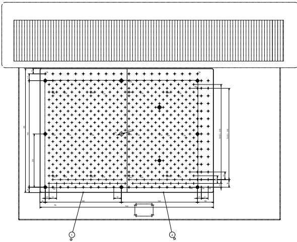
taban plakası K551191 CMM CRYSTA-Apex S7106 için
