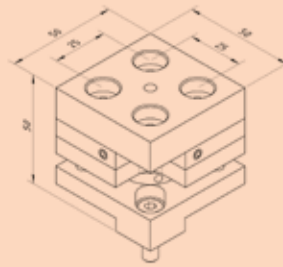
Parça No.: K551122 Ağırlık 290 g
