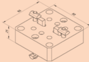
Parça No.: K551157 Ağırlık 460 g
