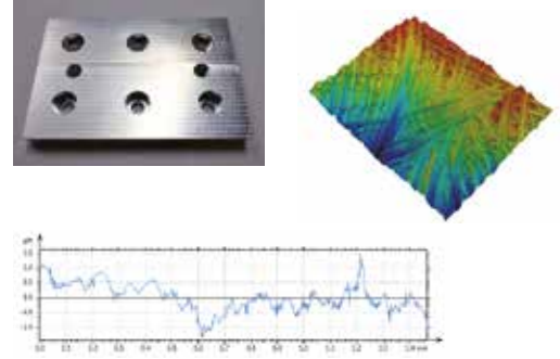
Metal işlenmiş yüzey (alüminyum)
