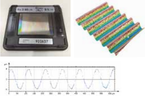
Pürüzlülük numunesi 3 µm
